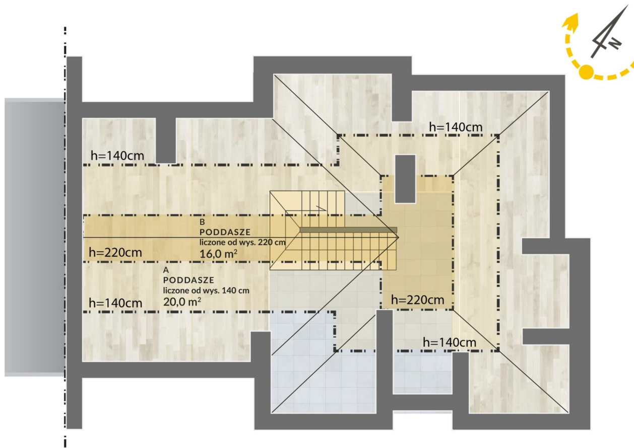
Rzut poddasza
