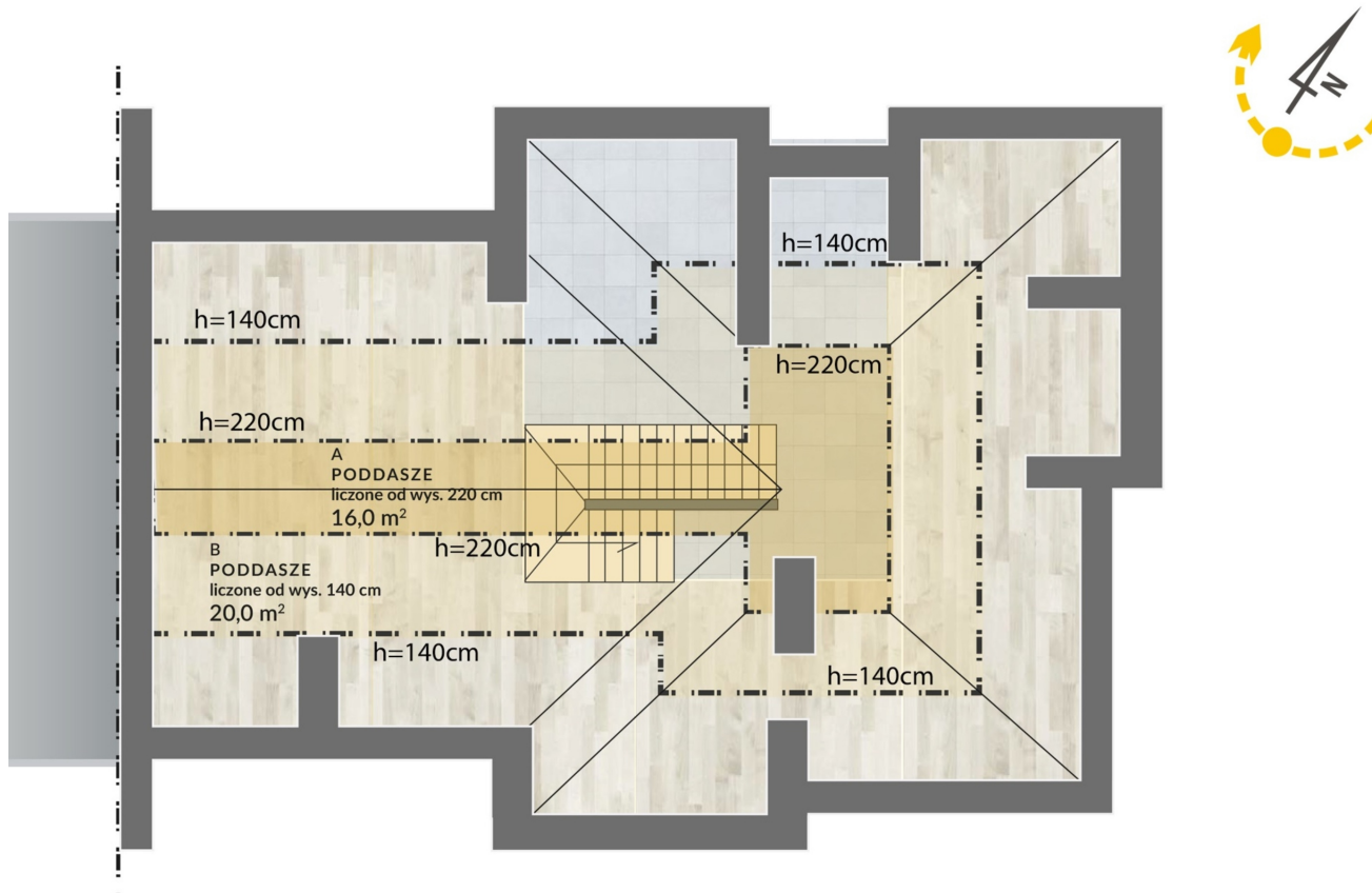
Rzut poddasza
